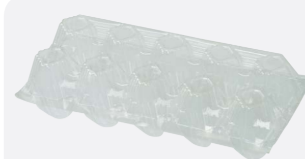
A1-10 材質 Material : PLA, PET 尺寸 Size : 234x109x66mm 數量 Quantity : 2000pcs 材積 Cu.ft. : 3.46'
