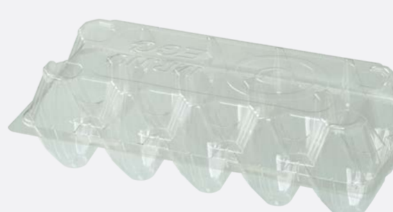
A2-10P 材質 Material : PLA, PET 尺寸 Size : 240x108x67mm 數量 Quantity : 1000, 800pcs 材積 Cu.ft. : 3.21', 3.21'
