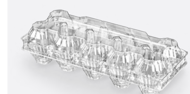
A2-10PJW 材質 Material : PLA, PET 尺寸 Size : 249x105x66mm 數量 Quantity : 600pcs 材積 Cu.ft. : 6.39'
