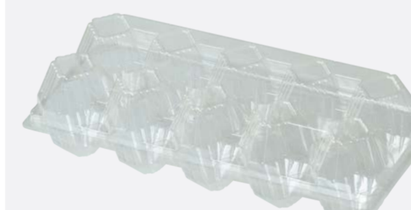
A2-10 材質 Material : PLA, PET 尺寸 Size : 240x108x68mm 數量 Quantity : 1200pcs 材積 Cu.ft. : 3.73'
