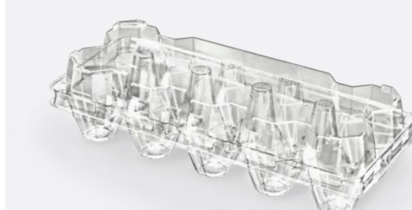
A2-10PCS 材質 Material : PLA, PET 尺寸 Size : 243x101x64mm 數量 Quantity : 700pcs 材積 Cu.ft. : 6.39'
