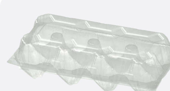
A1-8P 材質 Material : PLA 尺寸 Size : 228x110x66mm 數量 Quantity : 1200pcs 材積 Cu.ft. : 3.02'
